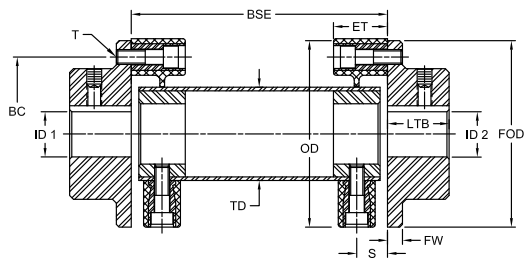
Model 6 (Zytel®)
