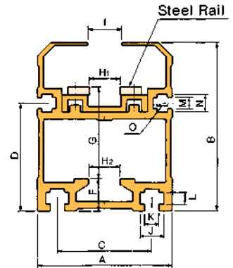
C2080VRP-R3LS
