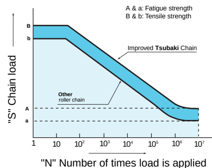
S-N Curve
