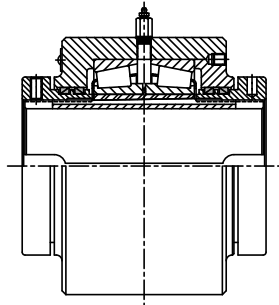
B-1 UNIT
