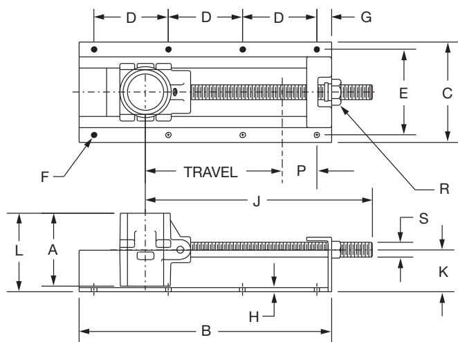
TYPE TUA
